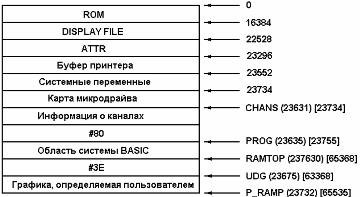
Рис. 1 Распределение памяти.
